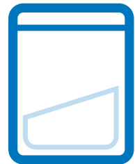
Kokain
